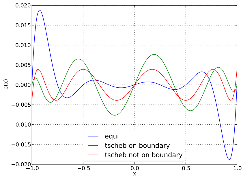
w_n(x) für Satz 8.10 mit n = 8
