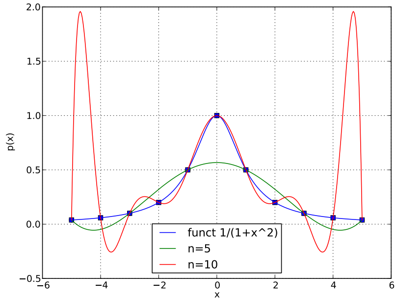
Beispiel von Runge mit äquidistanten Stützstellen n = 5, n = 10
