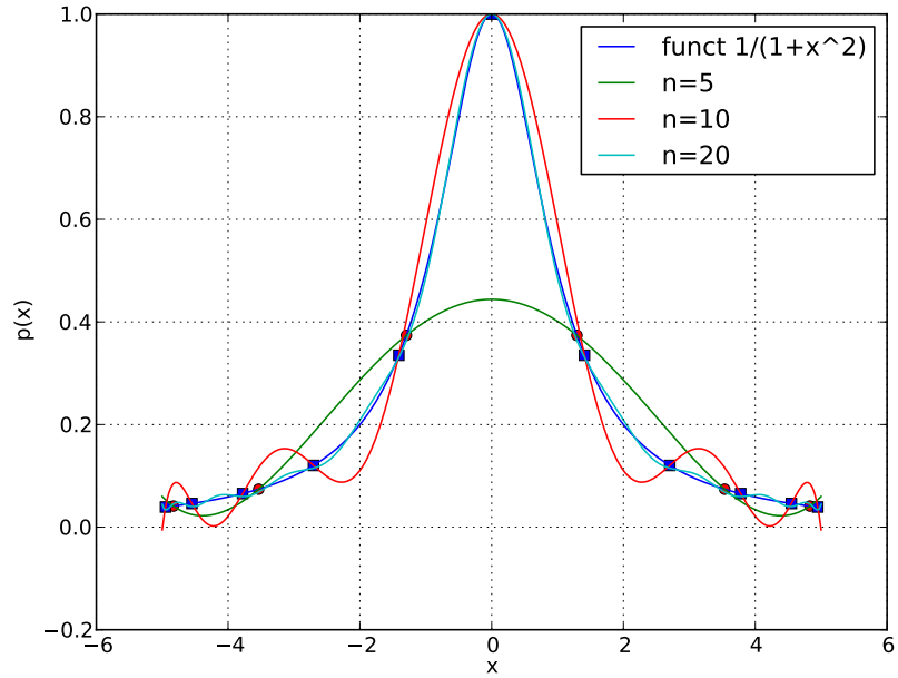
Beispiel von Runge mit Tschebyscheff Stützstellen n = 5 , n = 10 , n = 20
