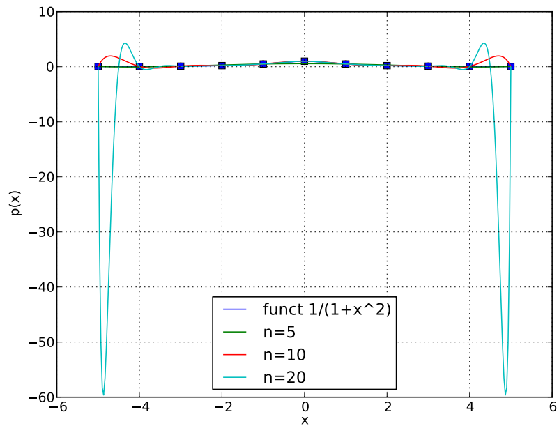
Beispiel von Runge mit äquidistanten Stützstellen n = 5 , n = 10 , n = 20
